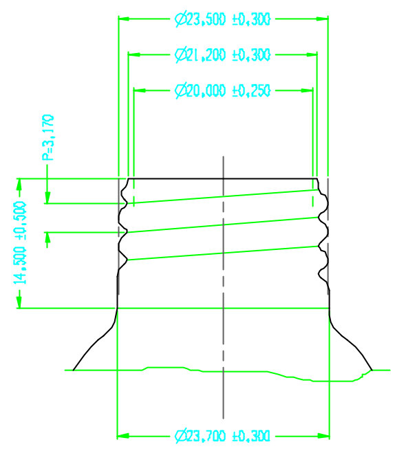
DETT. BOCCA Scala 2,5:1
